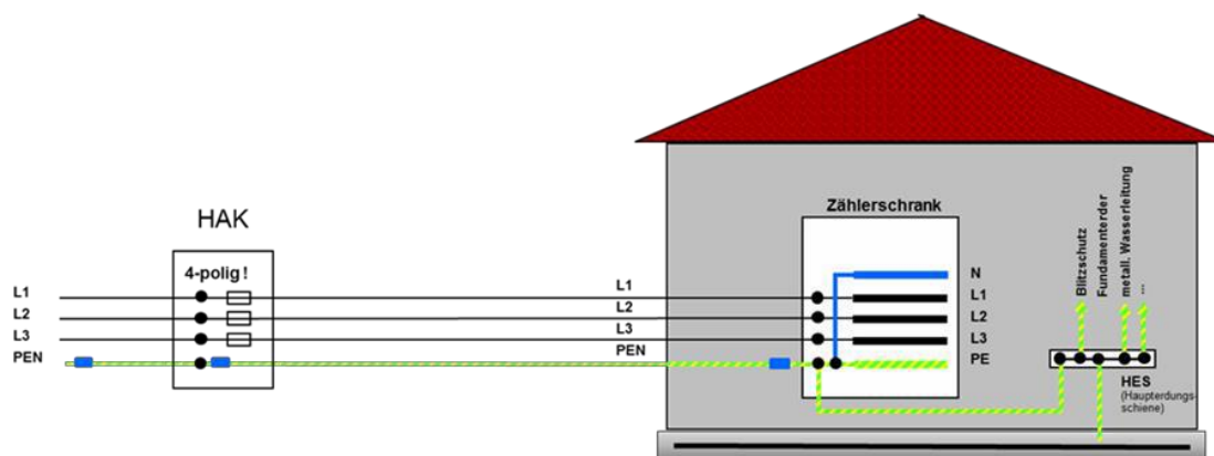
Abb. 16: Anschlussvariante bei TWN zur Außenanschlusstechnik (beispielhafte Darstellung)
